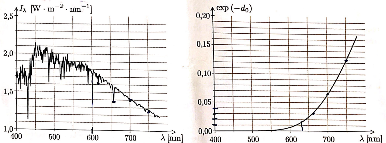
FIGURE 5 — À gauche : Spectre solaire hors de l'atmosphère terrestre. À droite : facteur d'atténuation spectrale \exp(-d_0)
