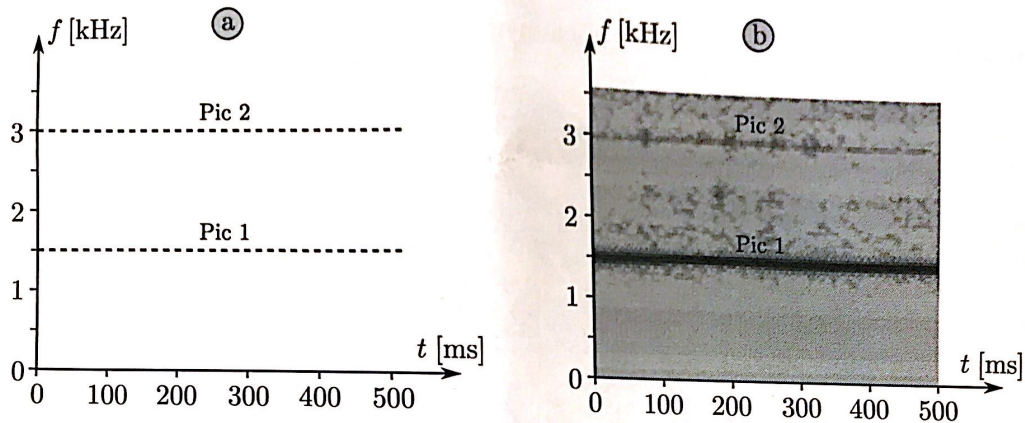
FIGURE 9 – Sonogramme d'un son sifflé tenu a) simplifié b) complet.
