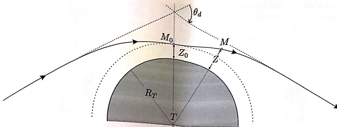
FIGURE 4 – Déviation d'un rayon lumineux par l'atmosphère terrestre.
