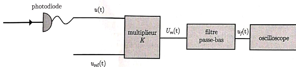
Figure 13 – Montage électronique pour réaliser le traitement du signal.
