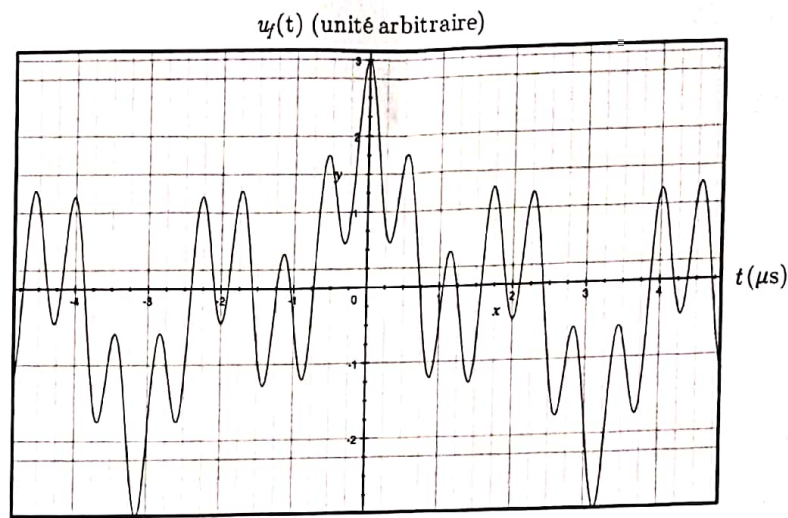
Figure 14 – Signal u_f(t) observé sur l'oscilloscope.
