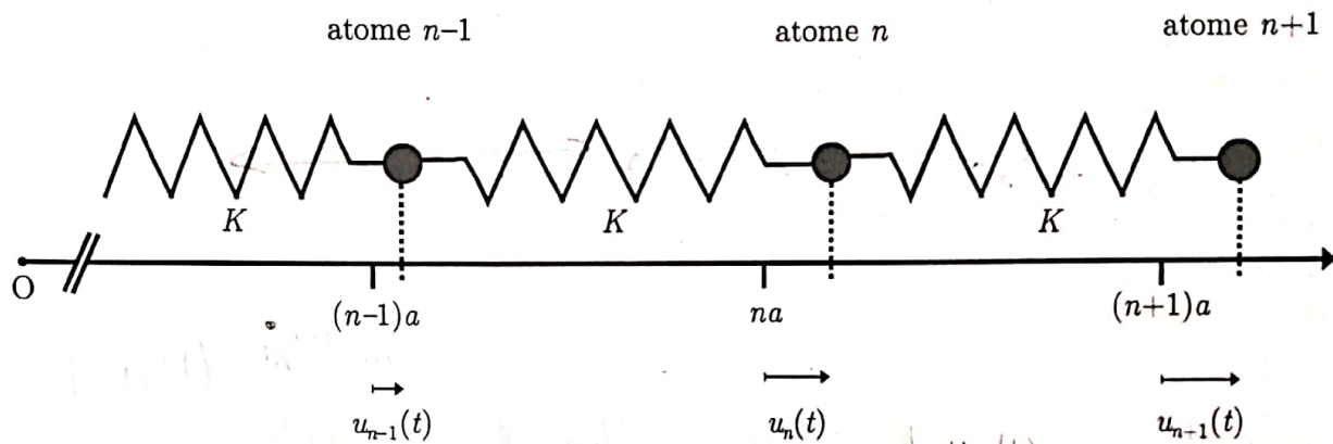
Figure 4 – Représentation du modèle unidimensionnel d'un cristal. Chaque atome est relié à deux voisins par un ressort de constante de raideur K et de longueur à vide a .
