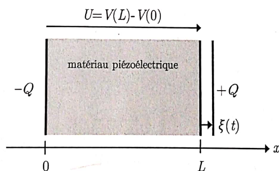
Figure 5 – Schéma d'un matériau piézoélectrique, limité par deux armatures conductrices situées en x = 0 et x = L et respectivement chargées -Q et +Q . L'armature placée en x = L est susceptible de se déplacer et son déplacement algébrique est noté \xi .
