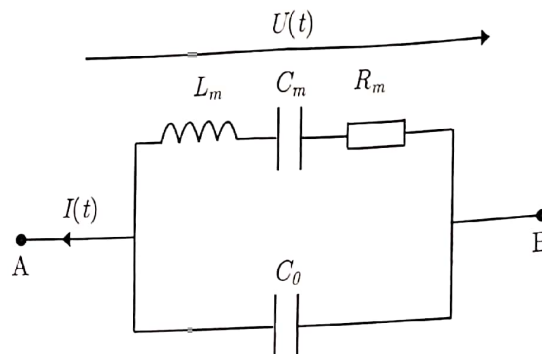
Figure 8 – Modélisation électrocinétique d'un transducteur piézoélectrique.
