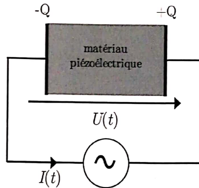
Figure 7 – Sollicitation d'un cristal piézoélectrique par une tension sinusoïdale.
