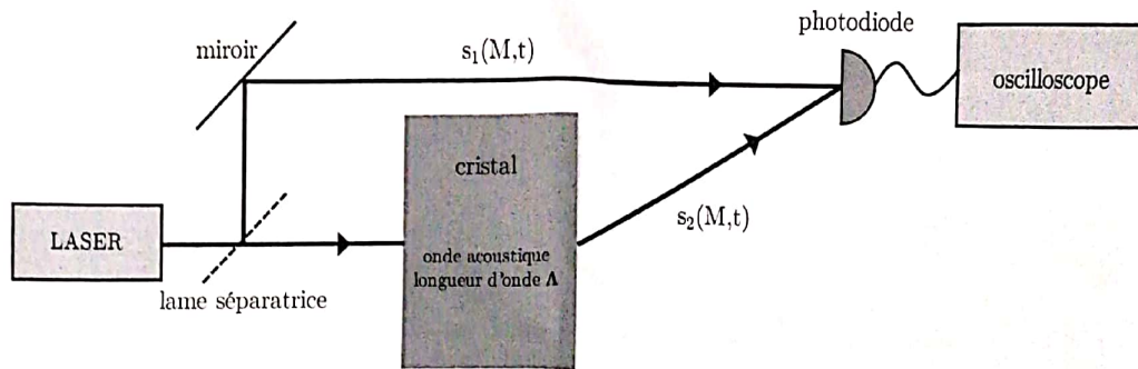
Figure 12 – Montage optique permettant de réaliser la superposition de deux ondes lumineuses.
