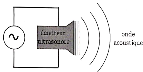
Figure 1 – Un émetteur ultrasonore connecté à une source de tension sinusoïdale émet une onde acoustique via la vibration d'un matériau piézoélectrique.
