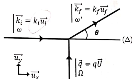
Figure 10 – Approche corpusculaire de l'interaction d'une onde électromagnétique avec une onde acoustique dans un cristal. Le vecteur d'onde et la pulsation sont rappelés pour chaque particule et quasi-particule.
