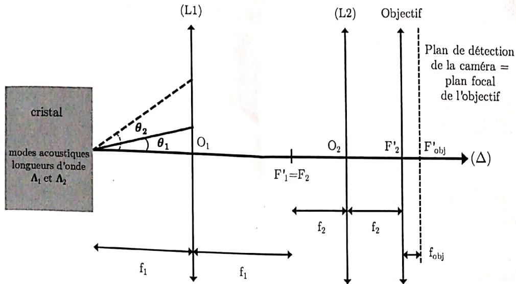
Figure 11 – Montage optique permettant la mesure des angles en sortie du cristal.
