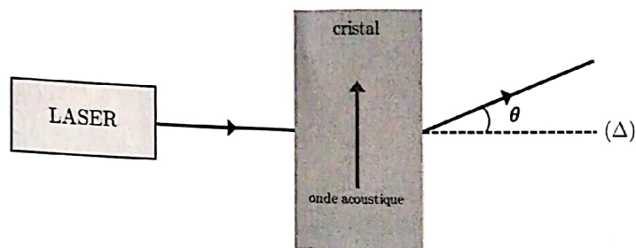
Figure 9 – Schéma de principe de l'utilisation d'un modulateur acousto-optique.
