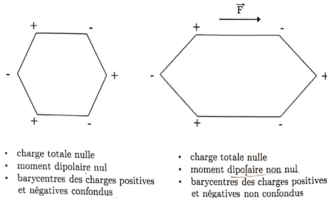
Figure 6 – Représentation schématique de la déformation d'une maille cristalline d'un matériau piézoélectrique et apparition d'un moment dipolaire.
