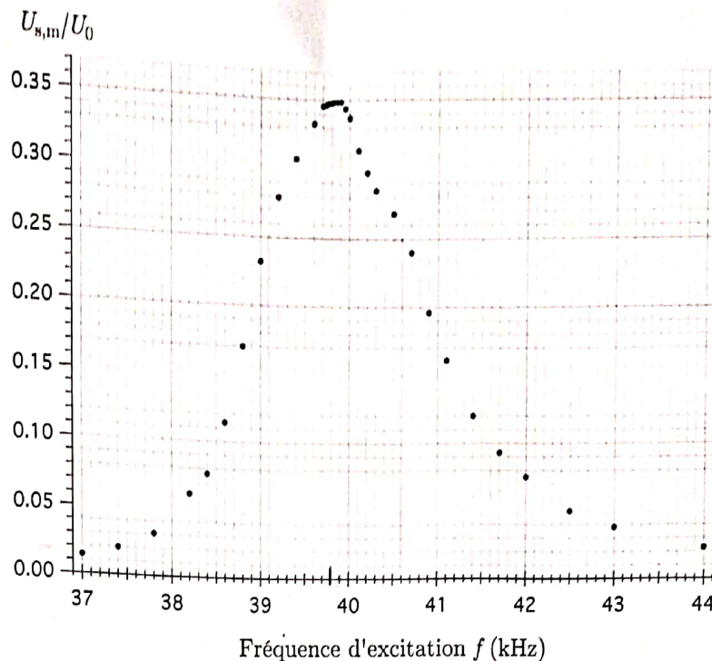
Figure 2 – Tracé de \frac{U_{s,m}}{U_0} en fonction de la fréquence d'excitation f .
