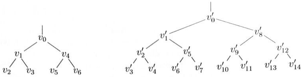
FIGURE 3 – Arbres binaires parfaits de hauteur 2 et de hauteur 3.
