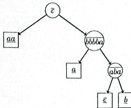
FIGURE 1 – Un exemple d'arbre discriminant : l'arbre \mathcal{T}_0
