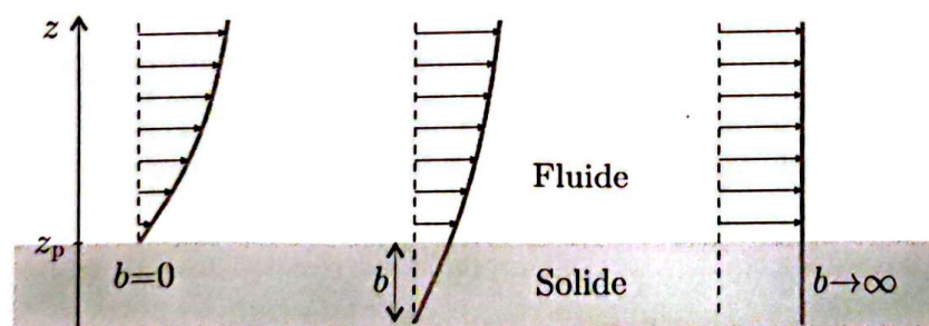
FIGURE 2 - Différentes conditions aux limites : glissement nul ( b = 0 ), partiel caractérisé par la longueur de glissement b > 0 , et total ( b \rightarrow \infty ) qui correspond à une condition de cisaillement nulle. Les flèches horizontales représentent le champ de vitesse dans le fluide.
