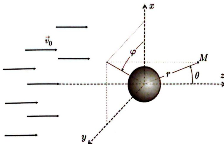
FIGURE 1 – Écoulement autour d'une boule et coordonnées sphériques.
