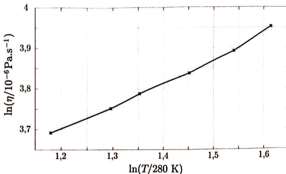
FIGURE 5 – Représentation graphique des mesures expérimentales de la viscosité de l'air pour différentes températures.
