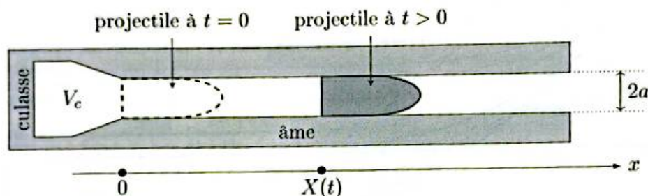
FIGURE 4 – Projectile dans un canon
