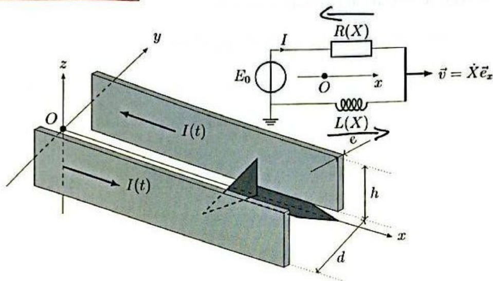
FIGURE 7 – Le propulseur d'un canon électromagnétique et son schéma équivalent
