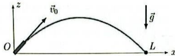
FIGURE 2 – Canon à eau en configuration de portée maximale
